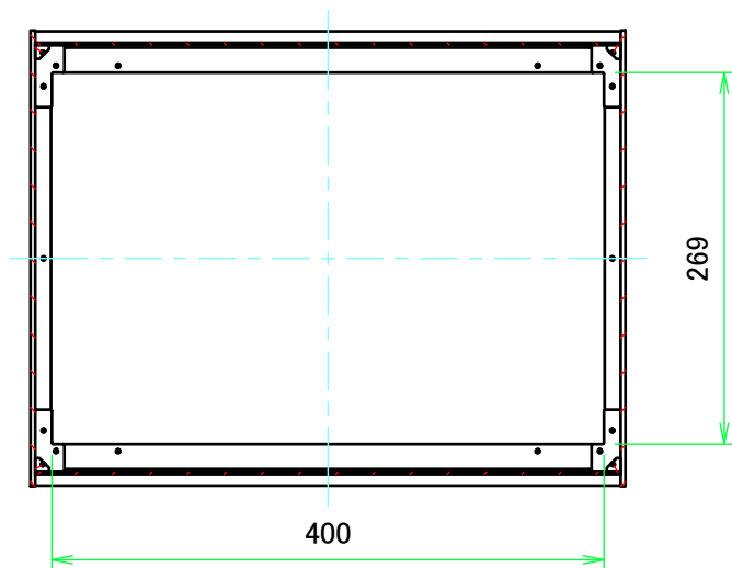
B-B ( 1 : 6 )
