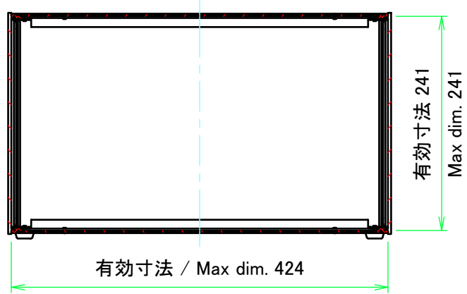
C-C ( 1 : 6 )
