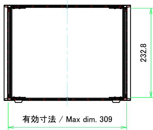
A-A ( 1 : 6 )
